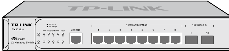
图 2-1 TL-SG3210 的前面板
